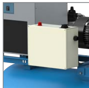
Přepínač hvězda-trojúhelník pro eliminaci proudových špiček a zatížení při rozběhu stroje.
